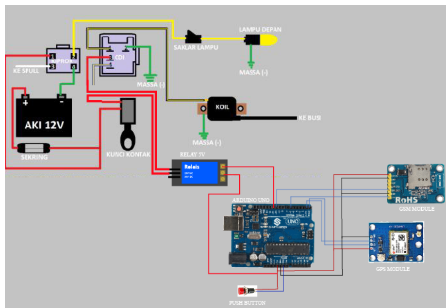
Fig. 1. Wiring diagram
